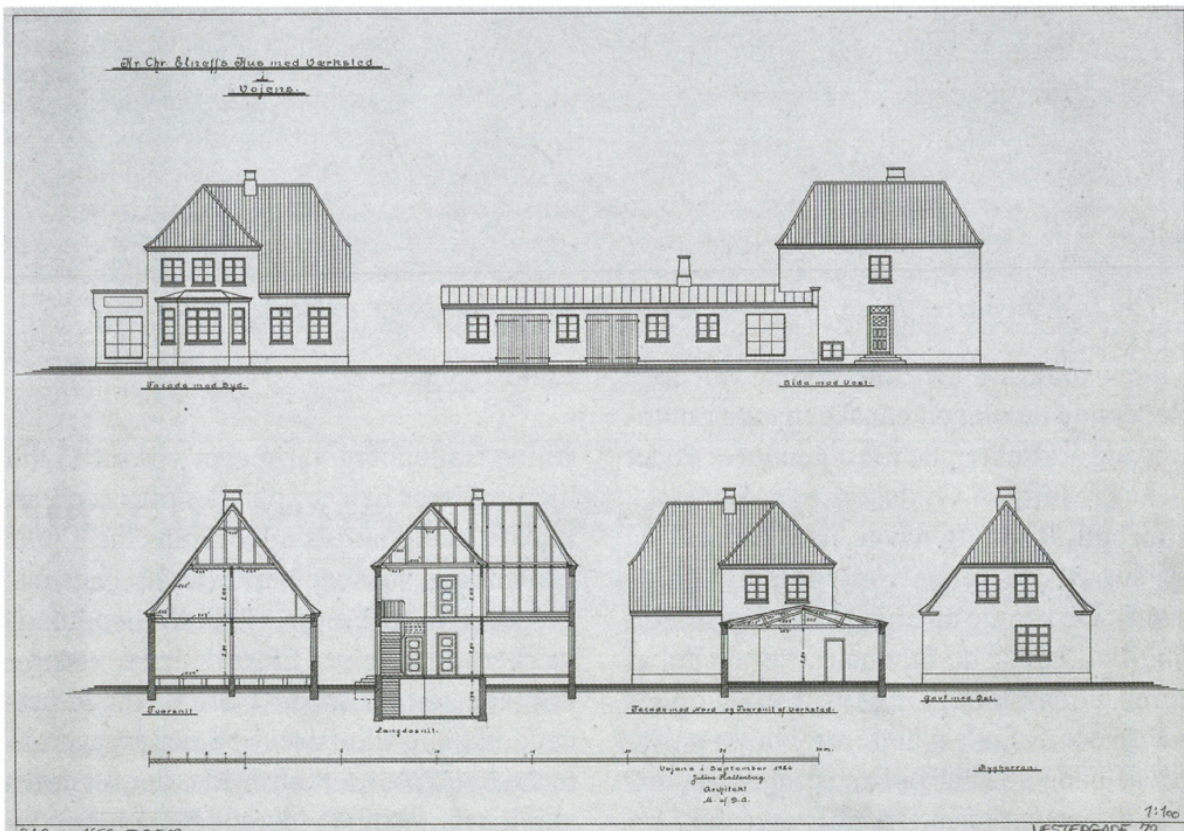
1926: Arkitekt J.P. Hallenbergs tegning af automobilmekaniker Chr. Elneffs hus, Vester-gade 72.
