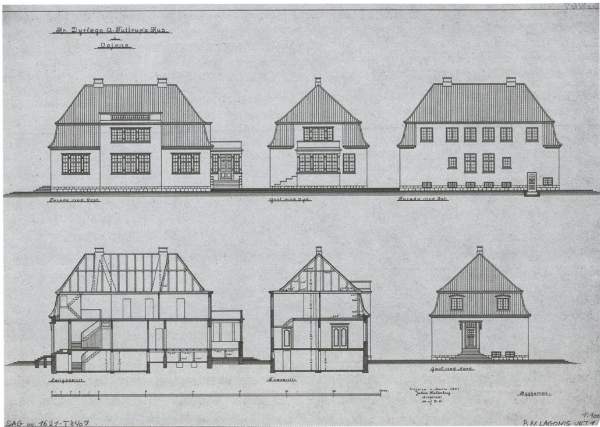
1927: Arkitekt J.P. Hallenbergs tegning af dyrlæge Anders Futtrups villa, Præstegårdsvej 5 (P. N. Lagonis Vej 1).
